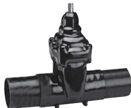
Серия 46/70 Клиновaя задвижка с длинными патрубками DN50-600 PN16 GP240GH С наружным покрытием PUR
